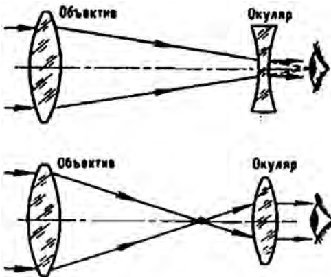
Рис. 3. Схема рефракторов Галилея (вверху) и Кеплера (внизу)
