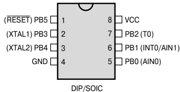
Рис. 1.2. Расположение выводов (вид сверху) моделей ATtiny11/11L
