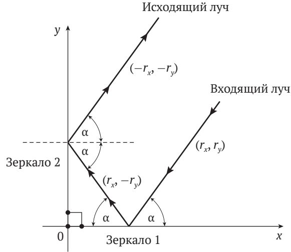
Рис. 1.3. Угловой отражатель на плоскости
