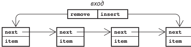
Рис. 1.2. Очередь в виде списка из четырех элементов
