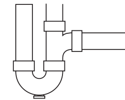
S-образный сифон с верхней вентиляцией
